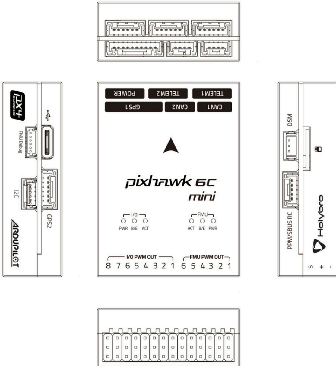
Pixhawk 6C Mini (Legacy)
